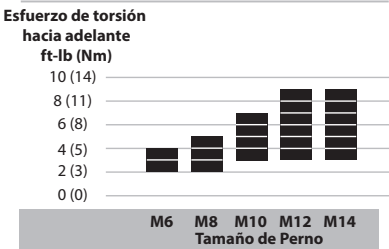
Figura A — Apriete Manual
