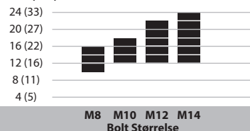
Figur B — Spændt til topnøglekraft
