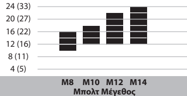
Προώθηση ροπής ft-lb (Nm)
