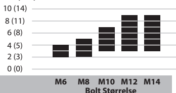
Figur A — Spændt til håndkraft
