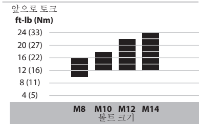
수치B — 렌치로 감기
