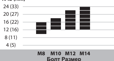
Фигура А — Затягане с гаечен ключ
