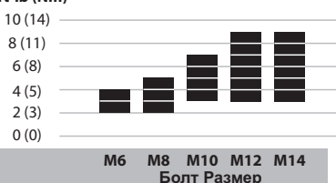
Фигура А — Затягане на ръка
