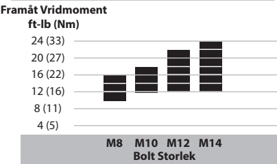
Figur B — Nyckelåtdragning
