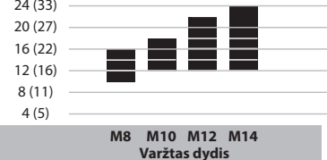
Persiūsti Sukimo momentas ft-lb (Nm)
