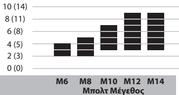
Προώθηση ροπής ft-lb (Nm)
